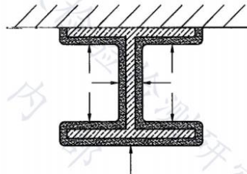
图 1 试件截面上涂层厚度测量点位置
